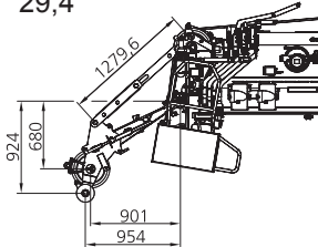
Lange Absteckung 29,4°
